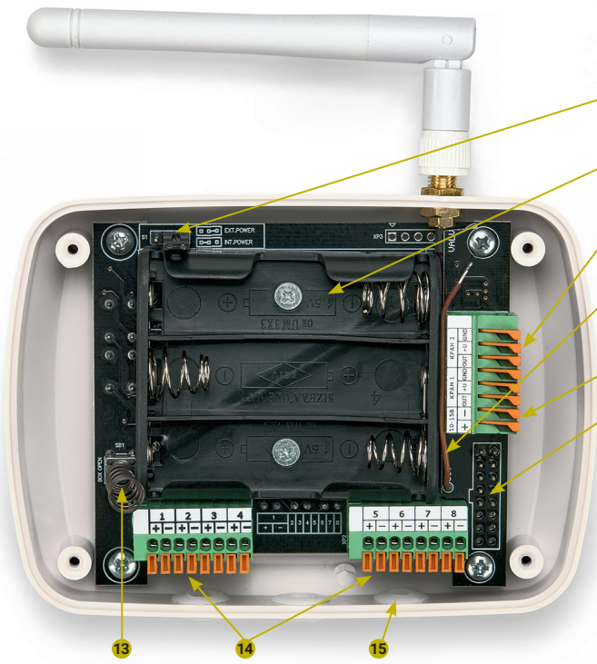
Фото 2. Блок управления HIDROLOCK Wi-Fi V2 со снятой задней крышкой
