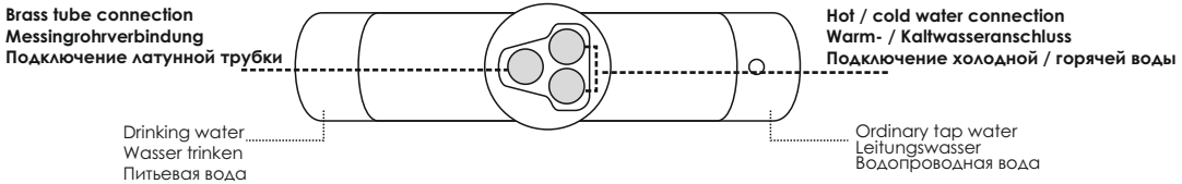
Mixer body, bottom view / Mixergehäuse, Ansicht von unten / Корпус смесителя, вид снизу
